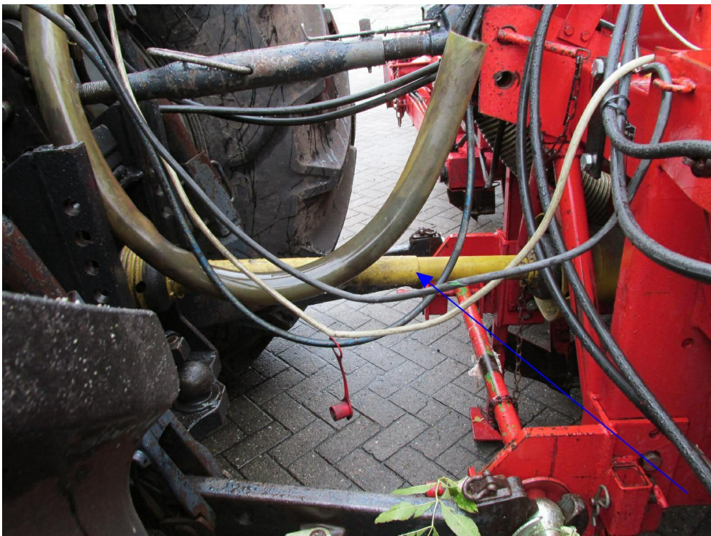
Bild 16: Dreipunktaufnahme mit Gelenkwelle
